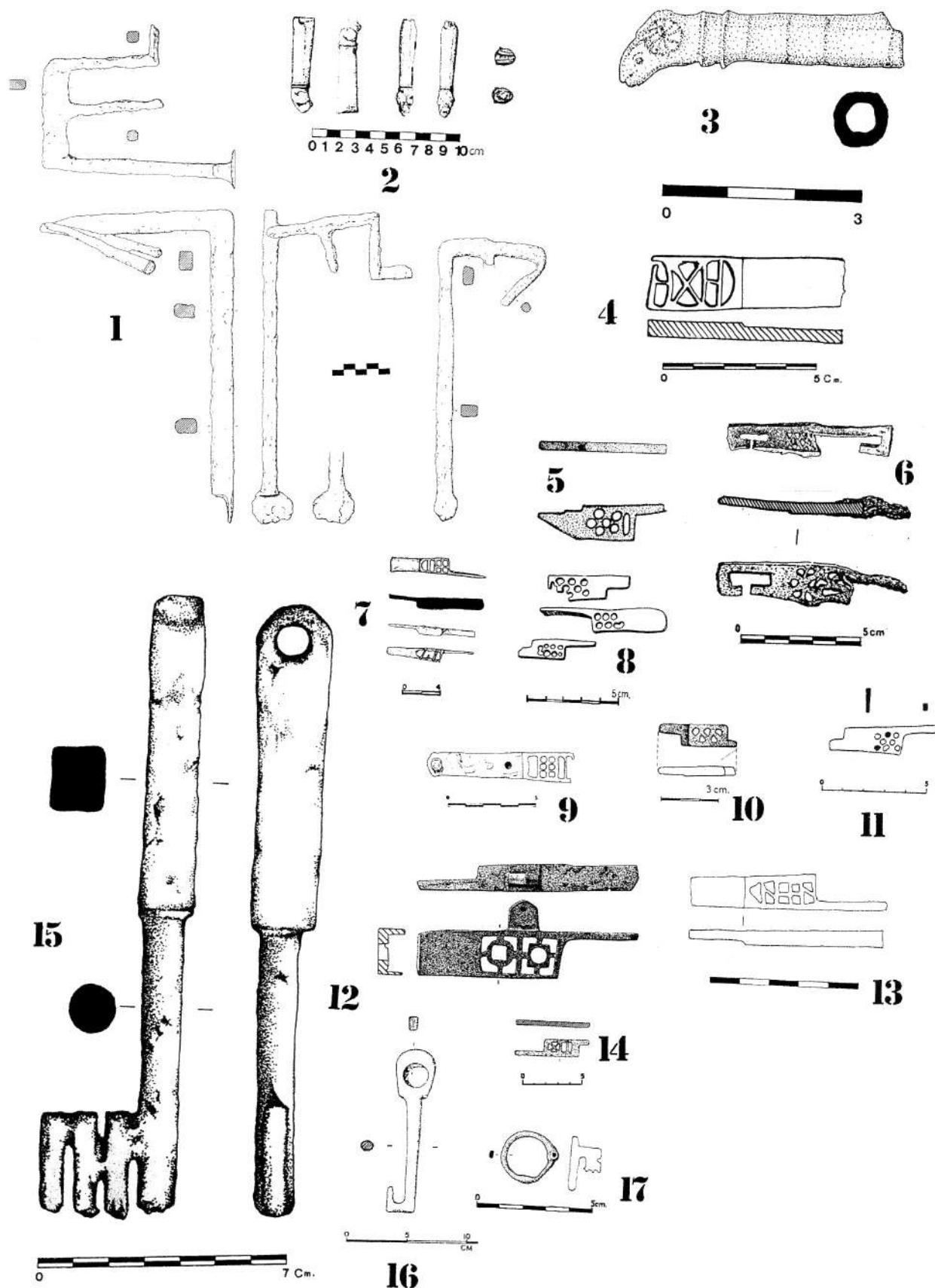
Figura 4: Llave de Giro (?), pestillos, mangos y llave-anillo. 1 – Getafe (sg. CABALLERO); 2 – Bilbilis (sg. CANCELA); 3 – Puente de la Olmilla (sg. AURRECOECHEA); 4 – Iuliobriga (sg. MORALES); 5 – El Saucejo (sg. FERNÁNDEZ y DEL AMO); 6 – Torres y Segobriga (sg. ALMAGRO); 7 – Arellano (sg. MEZQUÍRIZ); 8 – Torre Llauder (sg. RIBAS); 9 – Tiermes (sg. ARGENTE), 10 – Can Mercader (sg. ENRICH), 11 – Tolegassos (sg. CASAS y SOLER); 12 – Hondarribia (sg. URTEAGA); 13 – Bilbilis (sg. BUENO); 14 – Córdoba (sg. VARGAS); 15 – Iuliobriga (sg. FDEZ. IBÁÑEZ); 16 – Herrera de Pisuerga (sg. FDEZ. IBÁÑEZ); 17 – Sagunto (sg. LÓPEZ y DELAPORTE).
